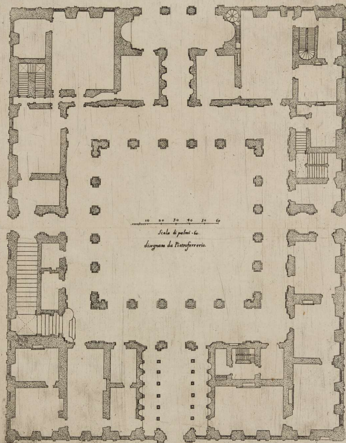
PIANTA DEL PALAZZO DI FARNESE FONDATA DA ANTONIO SANGALLO FAMOSO ARCHITETTO L. MDXXX.
