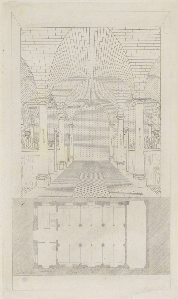
Massis erbauter Pferdestall auf dem Garten des H. O. H. Marshall's von Wangenheim zu Hannover. Gebaut durch L. v. L.
