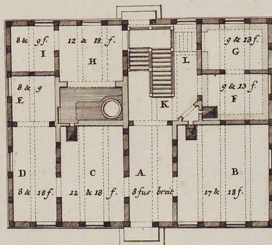
Grundriß der ersten Etage.
