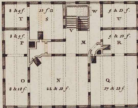
Grundriß der zweiten Etage.
