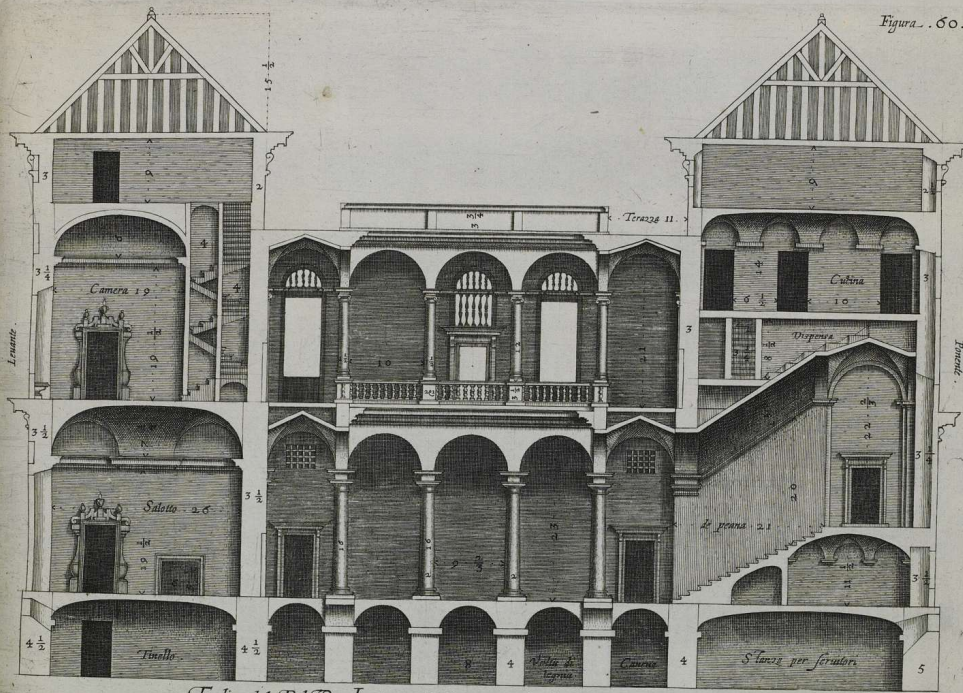
Taglio del Palazzo I. trauerfando tutto l'edifizio insieme il Cortile da leuante verso ponente.
